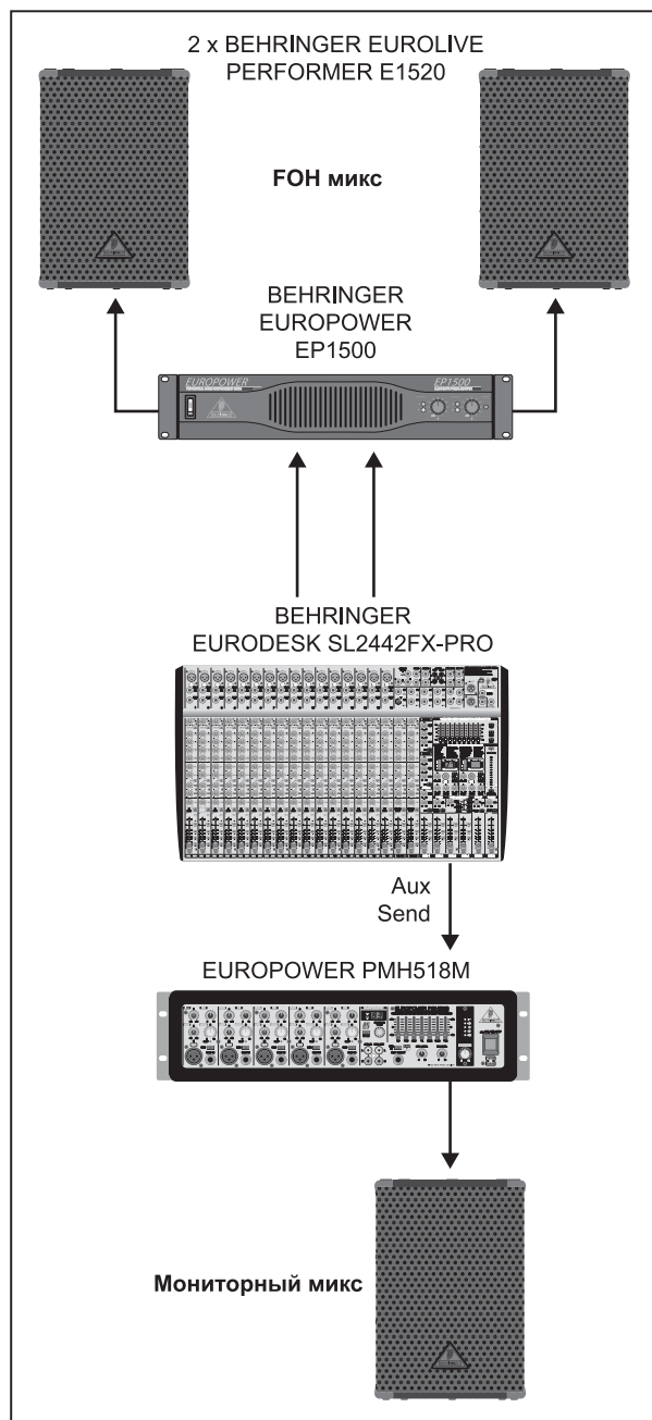
Рис. 5.2: Подключение PMH518M в качестве монитормого микшерного пульта
