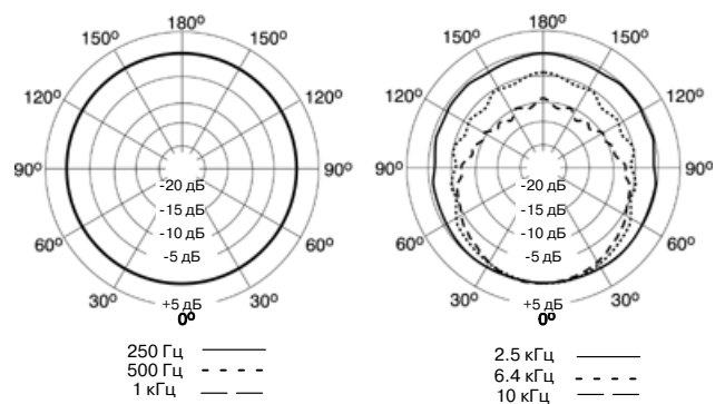
Круговая диаграмма направленности микрофона KSM141
