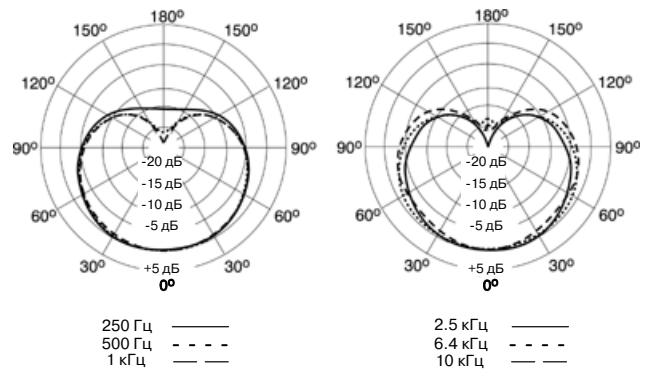
Кардиоидная диаграмма направленности микрофона KSM141
